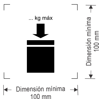
Figura 6-2. RIG apilables
